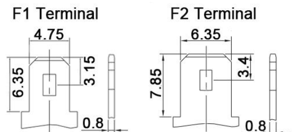
Złącze akumulatora
