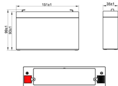
Wymiary
