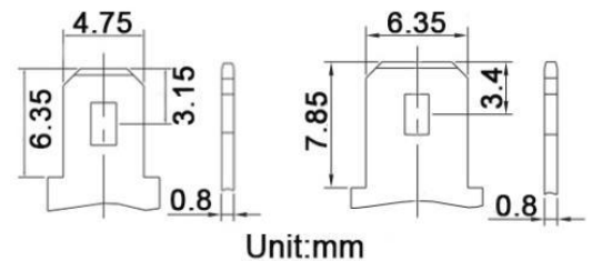
Złącze akumulatora
