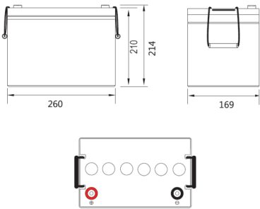
Wymiary
