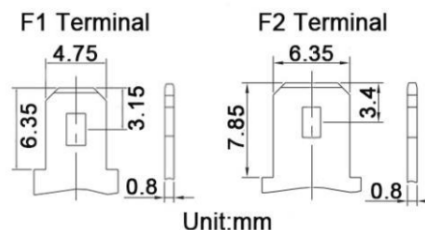
Złącze akumulatora
