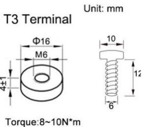
Złącze akumulatora
