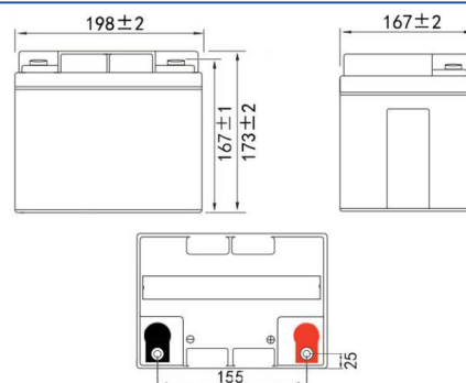
Wymiary
