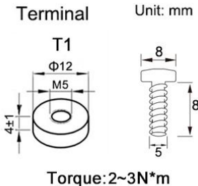
Złącze akumulatora
