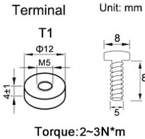
Torque: 2~3N*m
