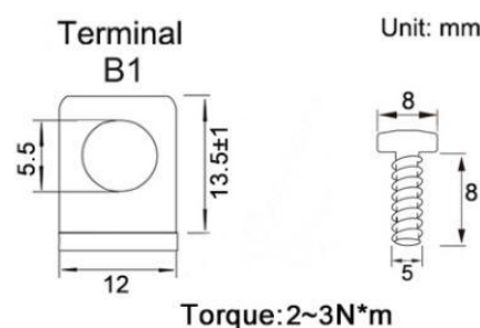
Złącze akumulatora
