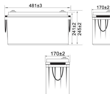
Wymiary
