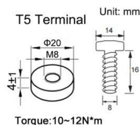
Złącze akumulatora
