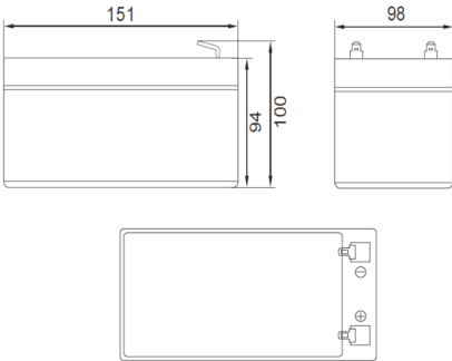
Wymiary
