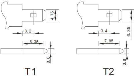
Złącze akumulatora
