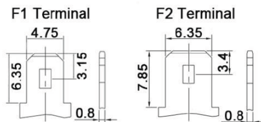
Złącze akumulatora
