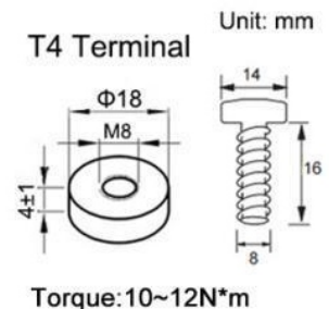
Złącze akumulatora
