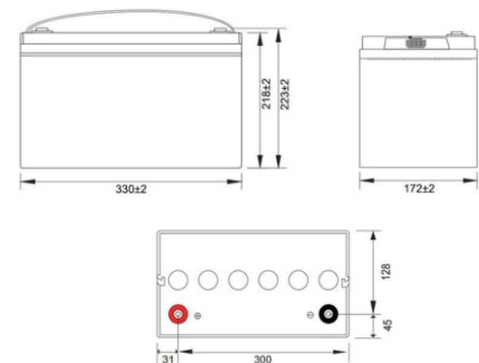
Wymiary
