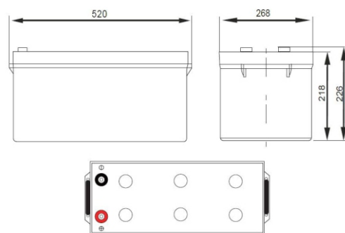
Wymiary
