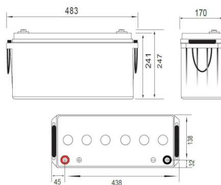
Wymiary
