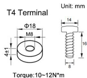
Złącze akumulatora
