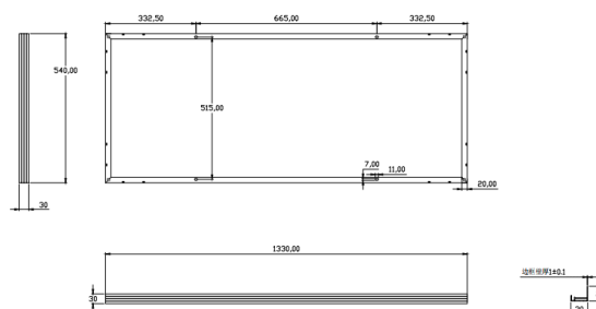
Wymiary
