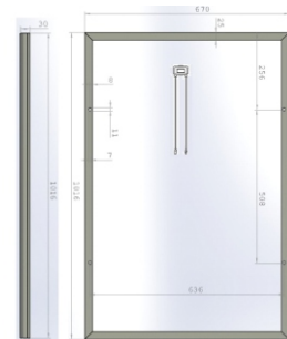
Wymiary
