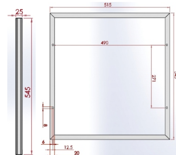
Wymiary
